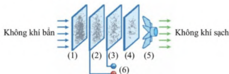
Hình 3. Sơ đồ máy lọc không khí
